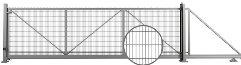
SCHIEBETOR MIT FÜLLUNG AUS VEGA 2D SUPER GITTERMATTEN, DIE AN DIE KONSTRUKTION ANGESCHRAUBT SIND – ANSICHT VOM GRUNDSTÜCK AUS.
